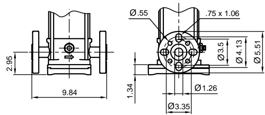
Flange 1-1/4" ANSI 300#
